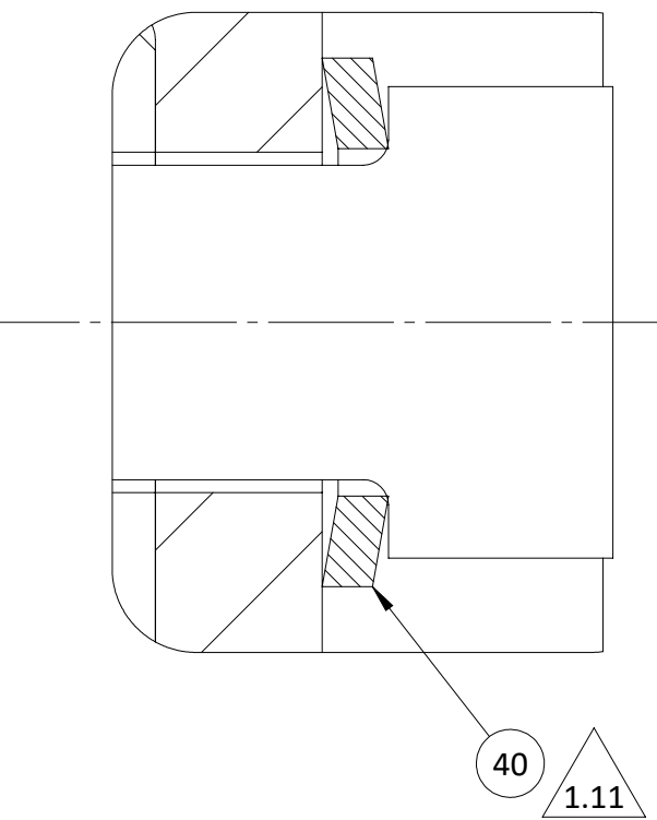
DETAIL Y SCALE 4 : 1
